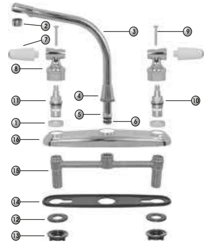
CARTUCHO CERÁMICO MODELO ACTUAL FIG. 8-IP
